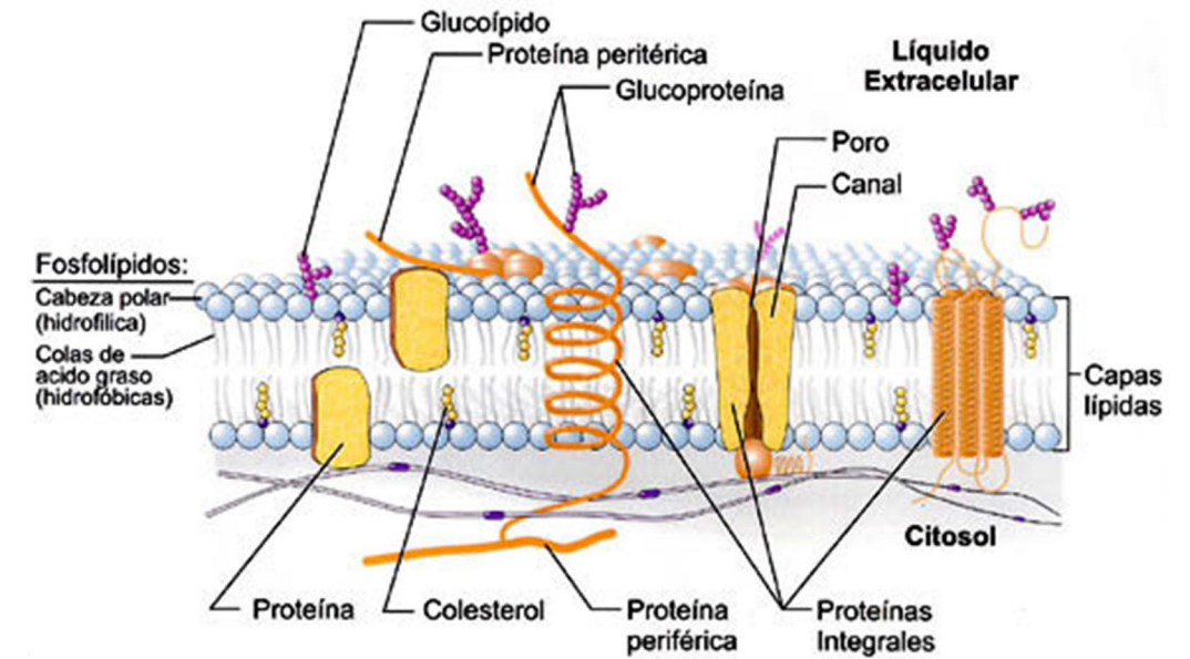
Figura 7 Estructura de la membrana celular
