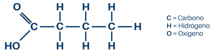
Figura 1 Estructura química de los lípidos simples
