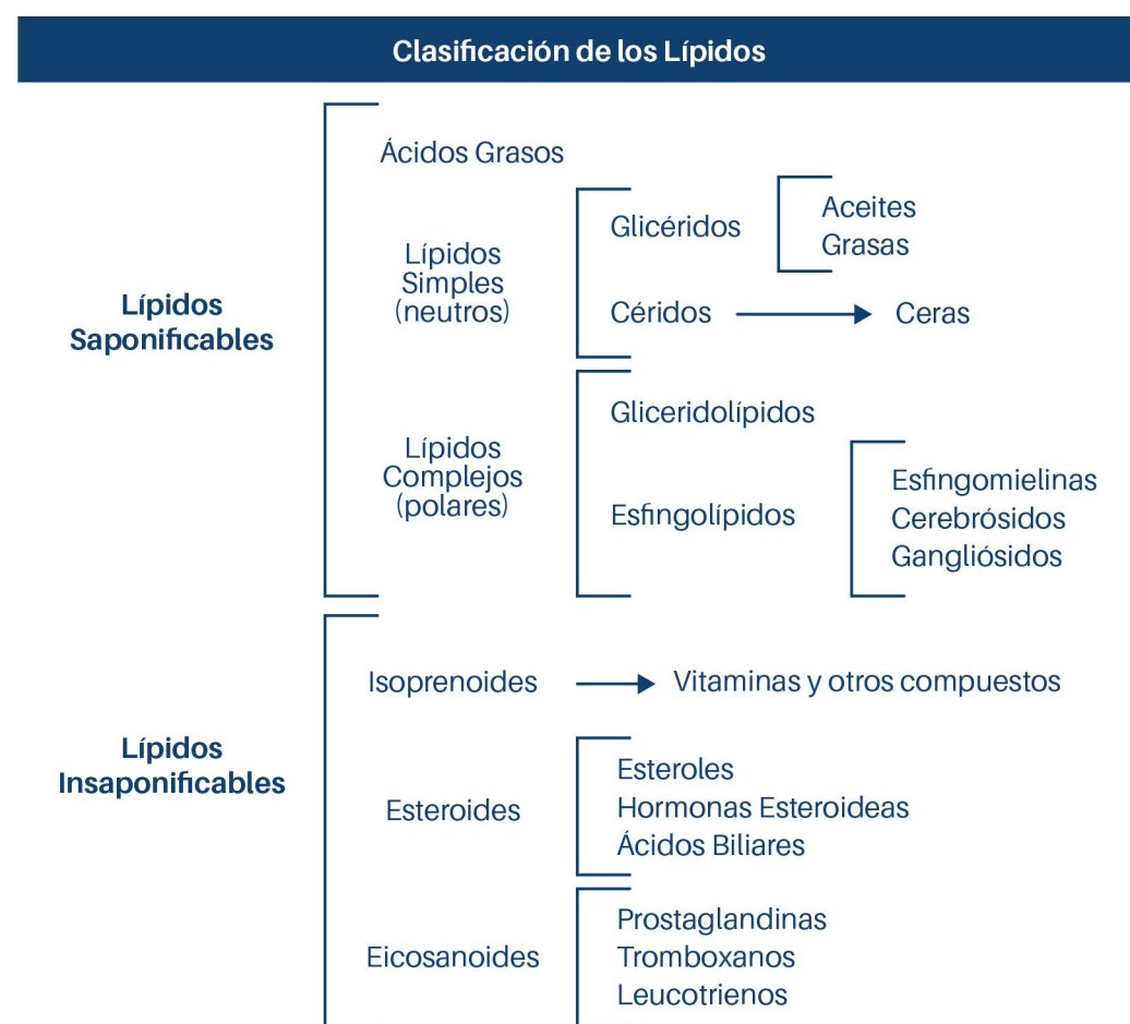
Figura 3 Clasificación actualizada de los lípidos
